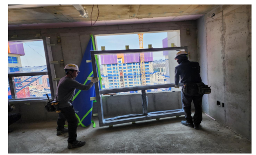
창호 설치 반드시 2인1조 이상으로하여 작업
