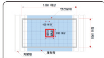
평면도 (제작기준)
