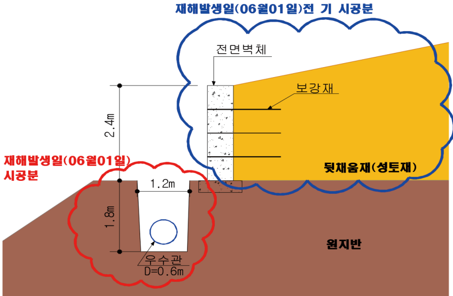
[사진1] 재해구간 시공현황
