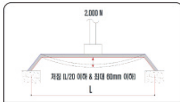
단면도 (성능기준: 처짐)
