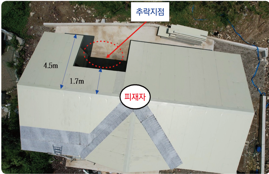
[사진1] 재해발생 현장전경
