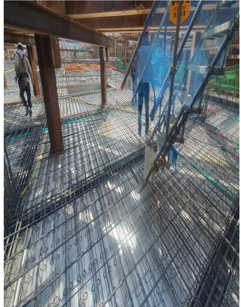
데크(철근) 설치구간 안전통로 미확보
