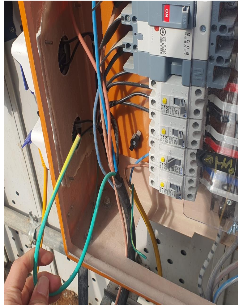
분전반 전선연결시 접지선 탈락
