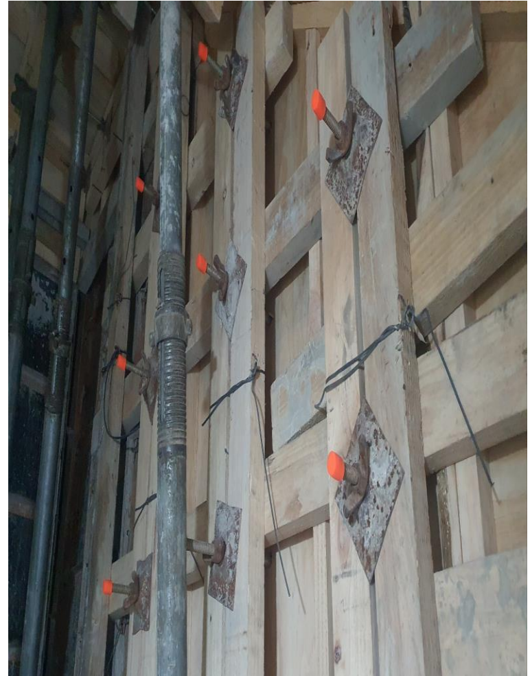
전단볼트 보양 캡 설치 우수
