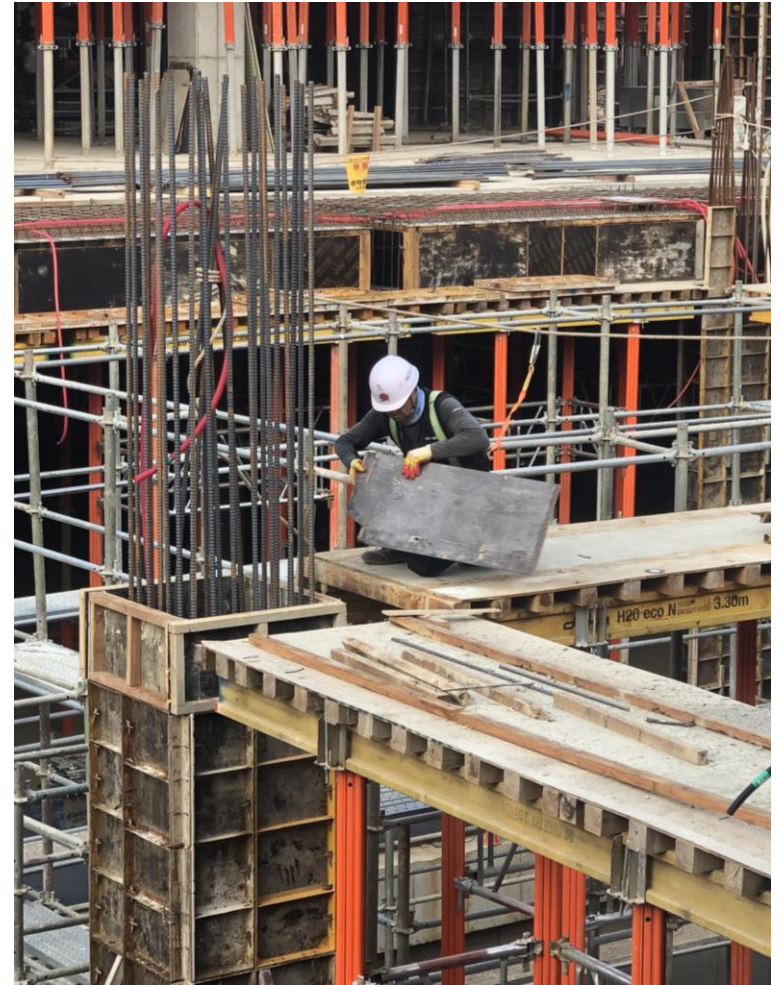
생명줄 설치 및 안전벨트 결속 우수
