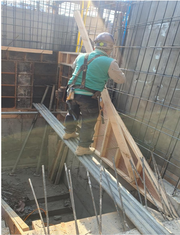
계단실 작업시 작업발판 설치 미흡
