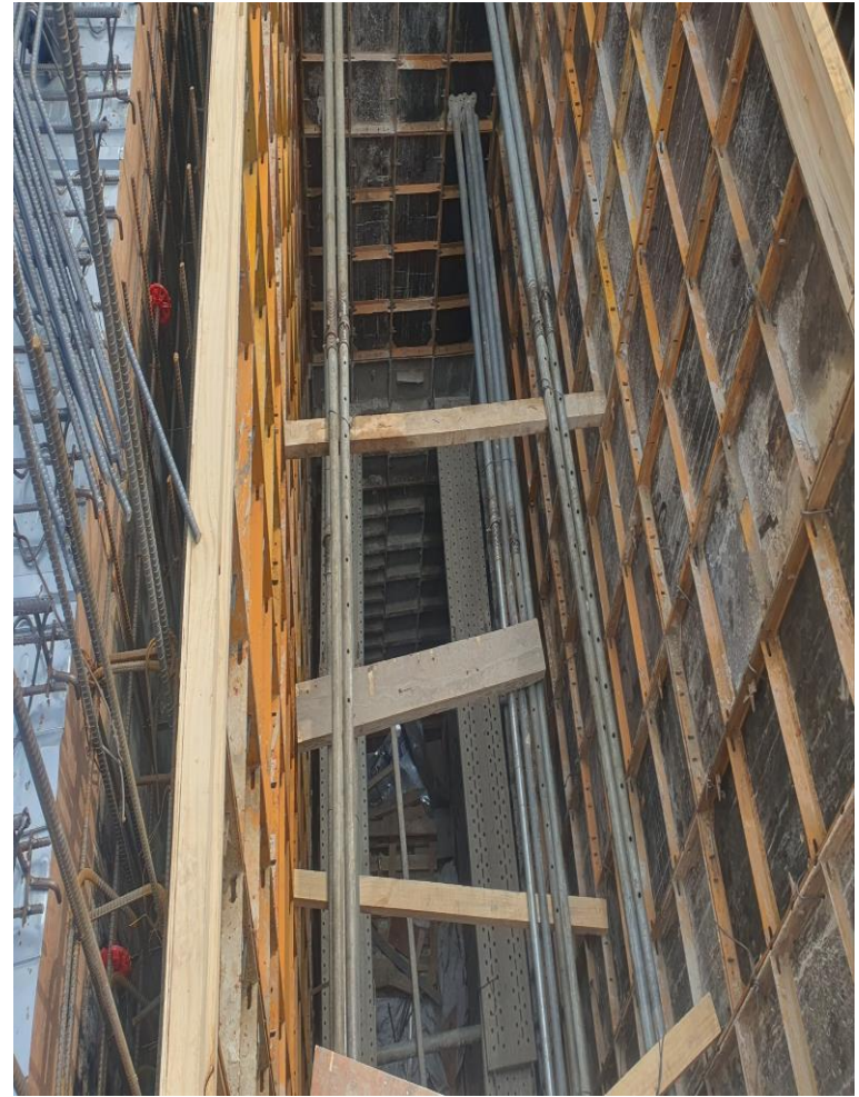
PIT구간 작업발판 설치 미흡 (발판 폭 불량 및 목재로 받침 사용)
