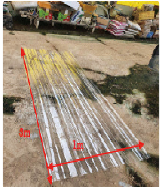
[사진2] 재해자와 함께 파단된 선라이트 및 교체중이던 선라이트 모습
